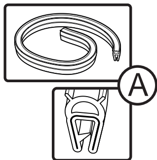
Perfil EPDM insertable EPDM clamping profile
