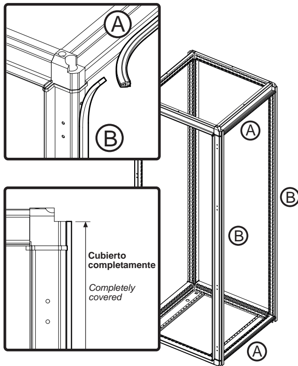
Perfil EPDM insertable EPDM clamping profile
