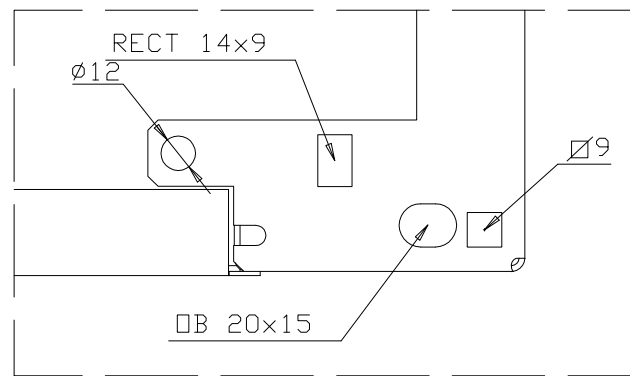
DETALLE X
