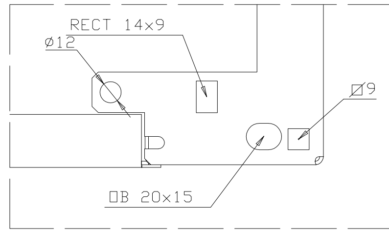
DETALLE X
