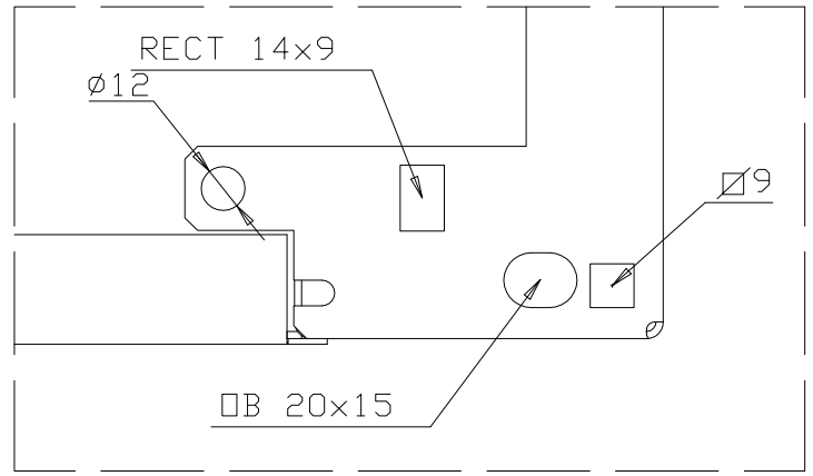
DETALLE X
