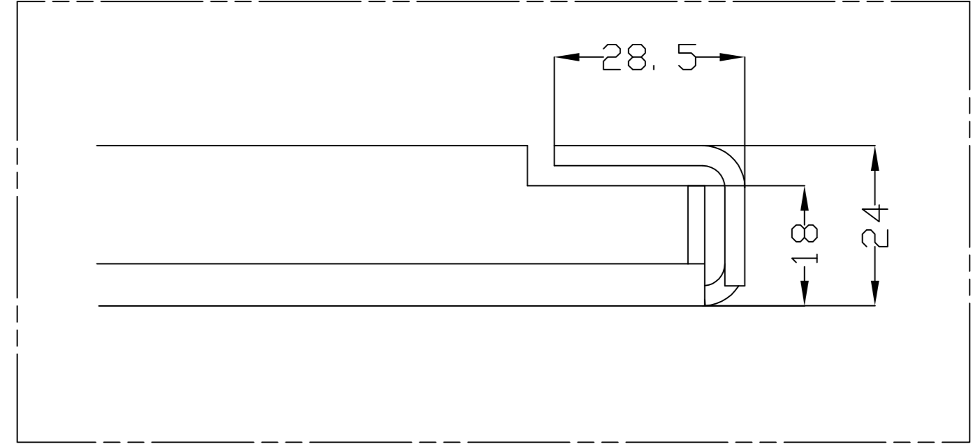
SEC. A-A
