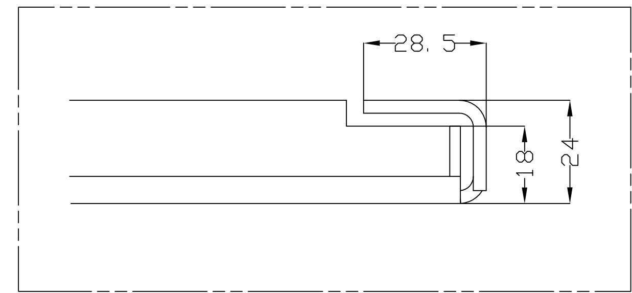
SEC. A-A
