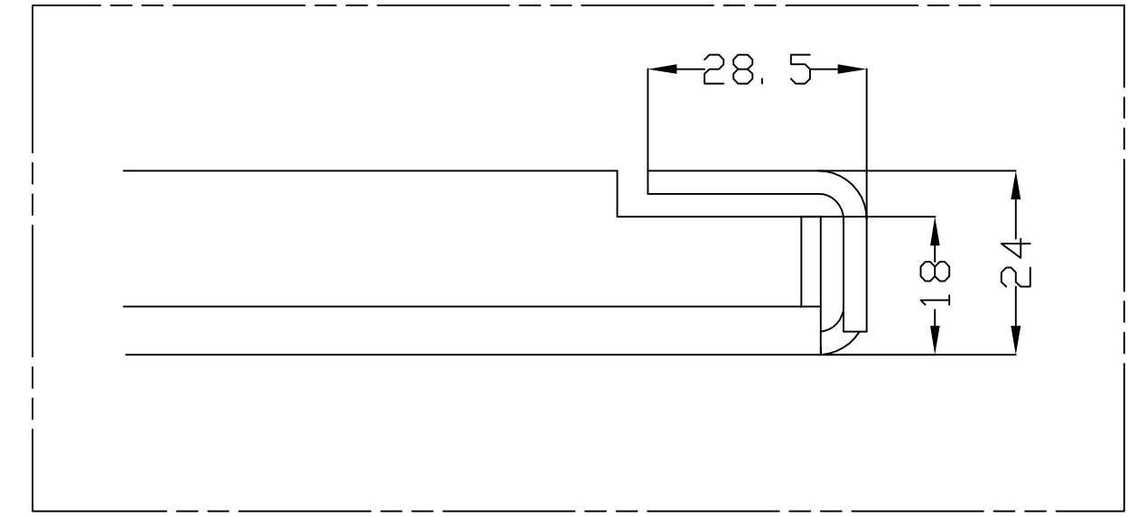
SEC. A-A
