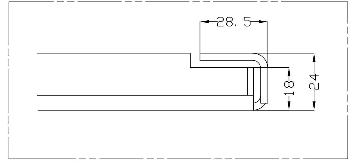
SEC. A-A
