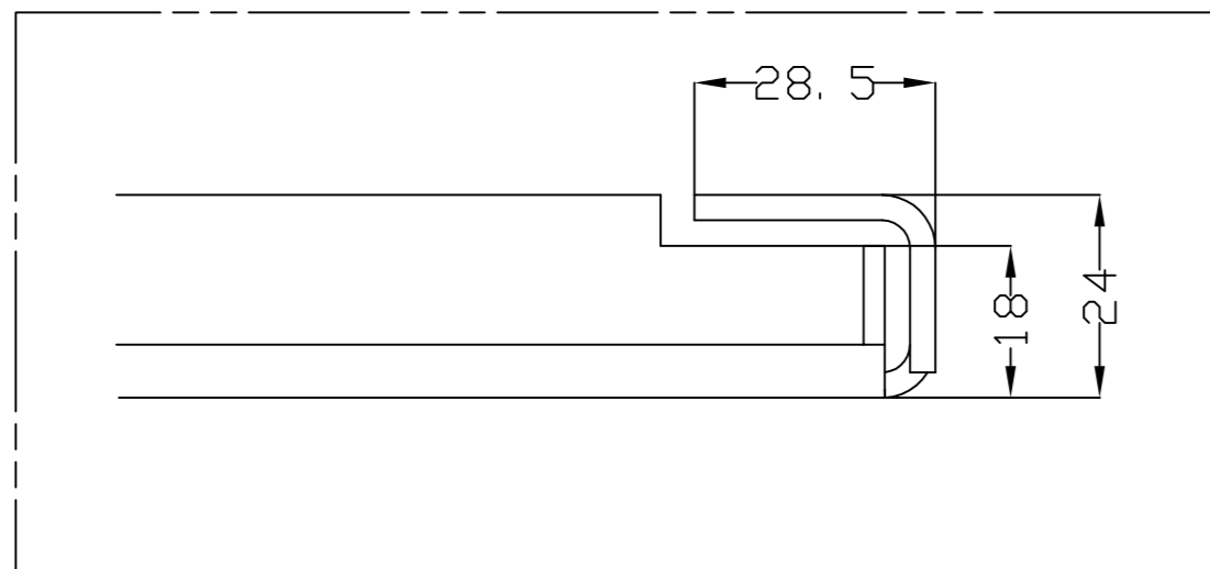
SEC. A-A
