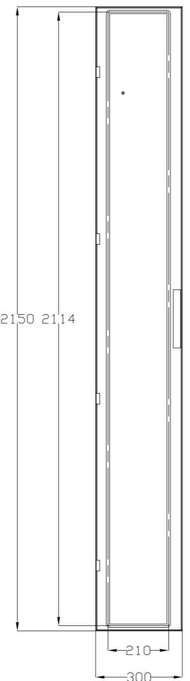
VISTA POSTERIOR PUERTA DOOR REAR VIEW
