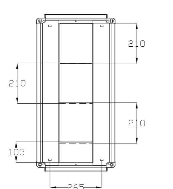
VISTA INFERIOR BOTTOM VIEW
