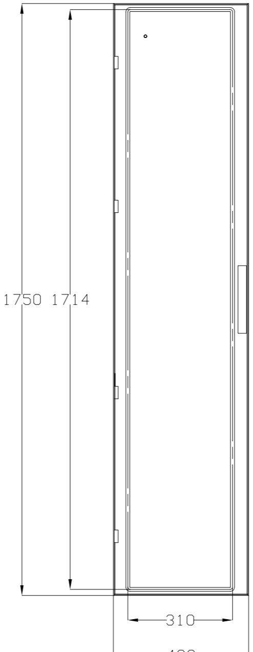
VISTA POSTERIOR PUERTA DOOR REAR VIEW
