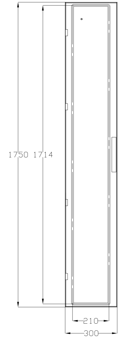
VISTA POSTERIOR PUERTA DOOR REAR VIEW
