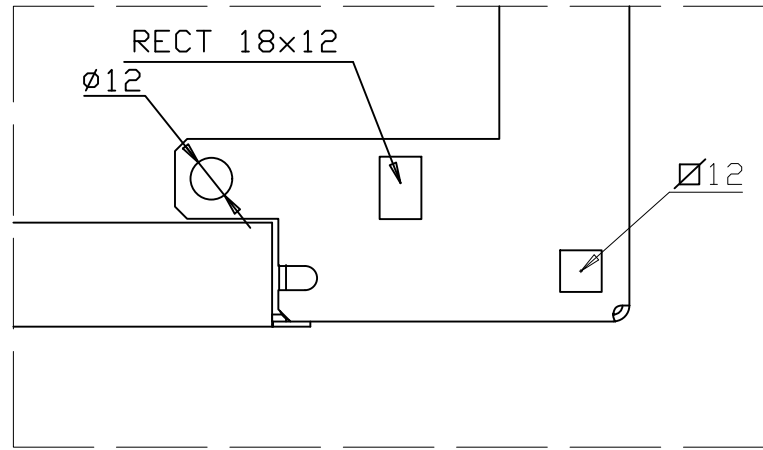
DETALLE X
