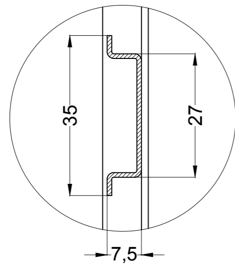
DETALLE A
