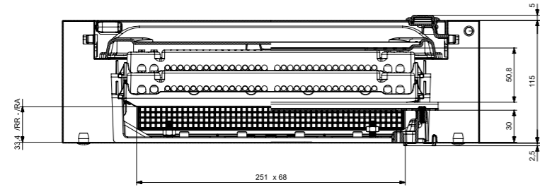
CORTE N-P-R-S
