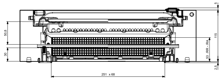
CORTE A-B-C-D
