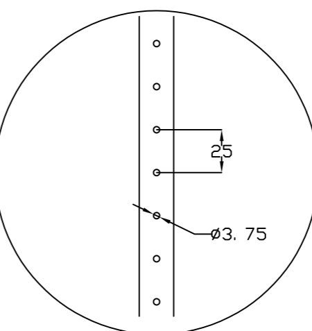
DETALLE DEL REFUERZO PROFILE DETAIL
