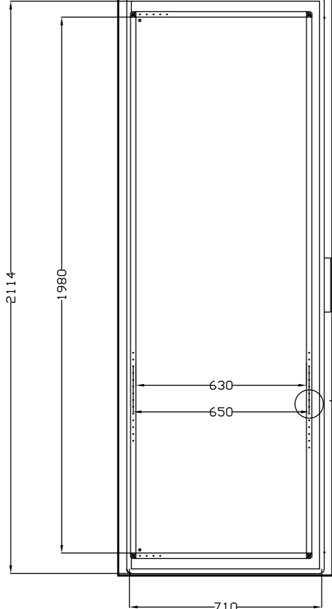
VISTA POSTERIOR PUERTA DOOR REAR VIEW
