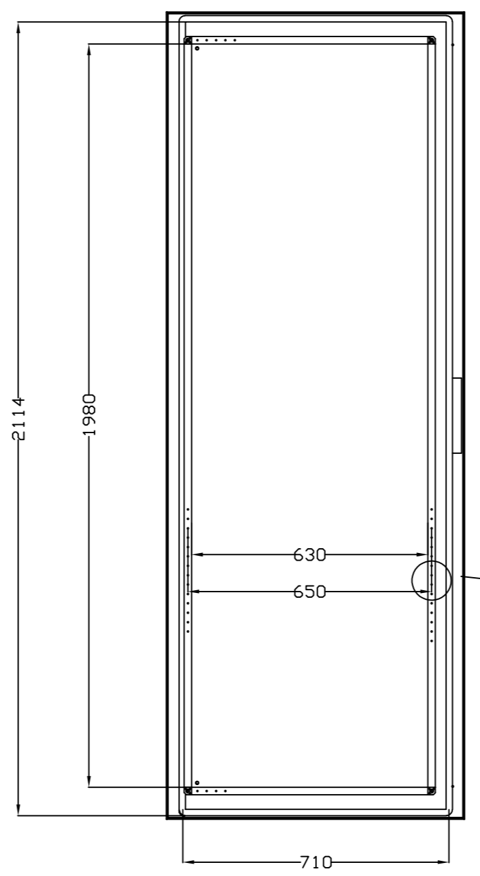
VISTA POSTERIOR PUERTA DOOR REAR VIEW
