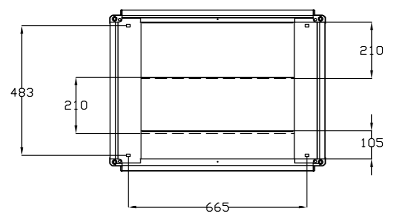
VISTA INFERIOR BOTTOM VIEW
