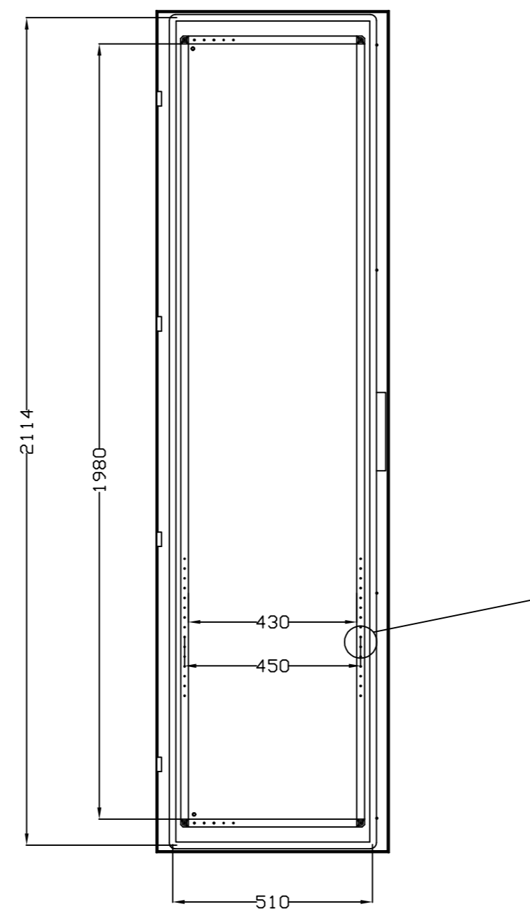
VISTA POSTERIOR PUERTA DOOR REAR VIEW
