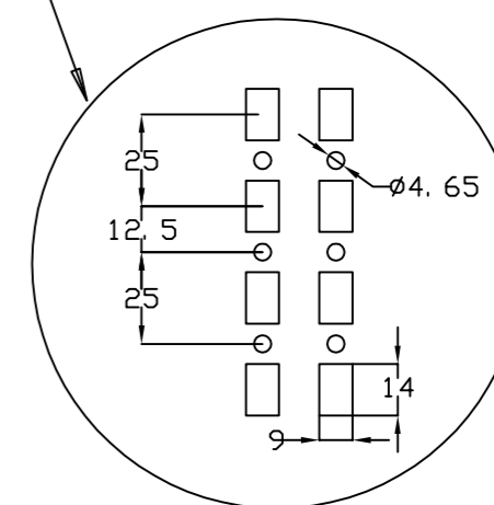
DETALLE DEL PERFIL PROFILE DETAIL
