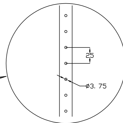
DETALLE DEL REFUERZO PROFILE DETAIL
