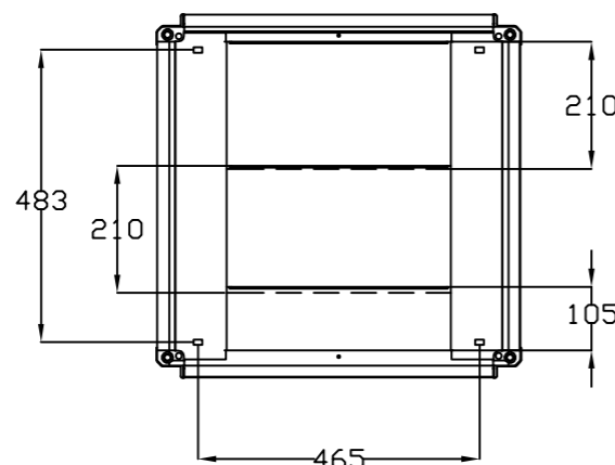
VISTA INFERIOR BOTTOM VIEW
