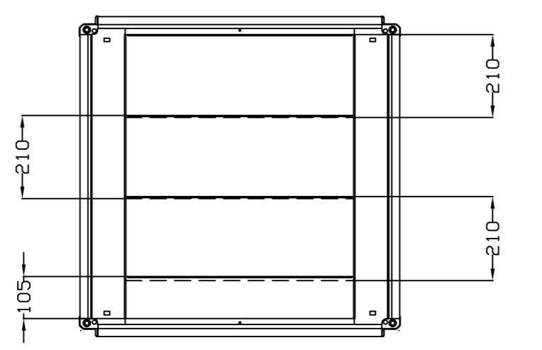
VISTA INFERIOR BOTTOM VIEW
