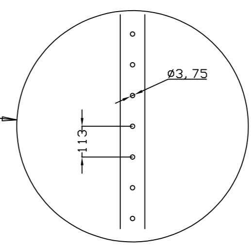
DETALLE DEL REFUERZO PROFILE DETAIL
