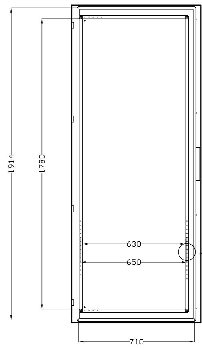
VISTA POSTERIOR PUERTA DOOR REAR VIEW
