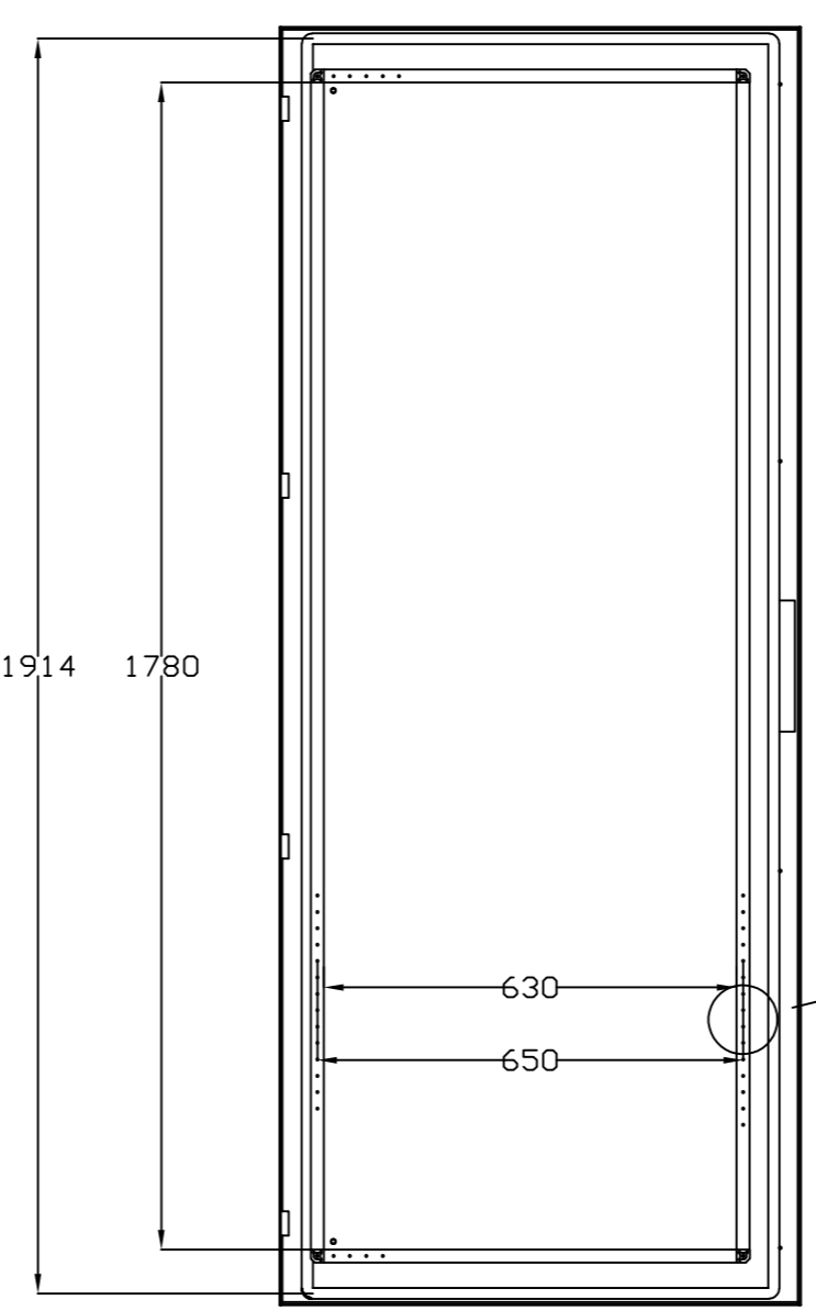
VISTA POSTERIOR PUERTA DOOR REAR VIEW
