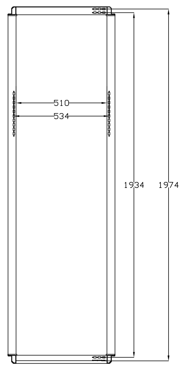
SEC. A-A
