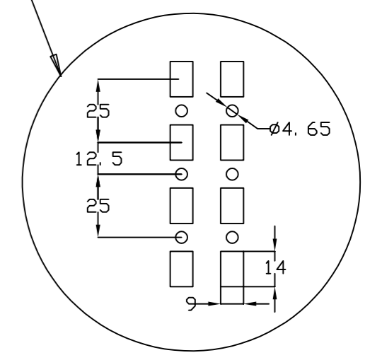
DETALLE DEL PERFIL PROFILE DETAIL
