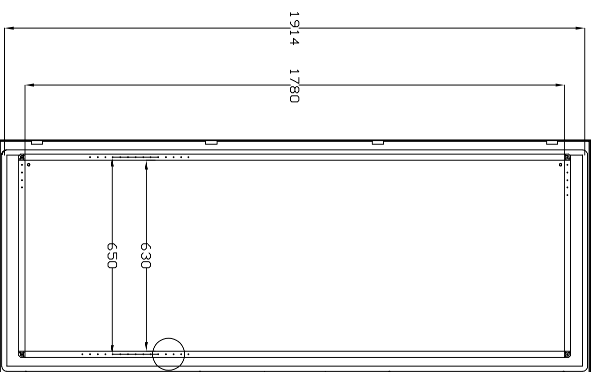
VISTA POSTERIOR PUERTA DOOR REAR VIEW
