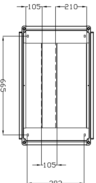
VISTA INFERIOR BOTTOM VIEW
