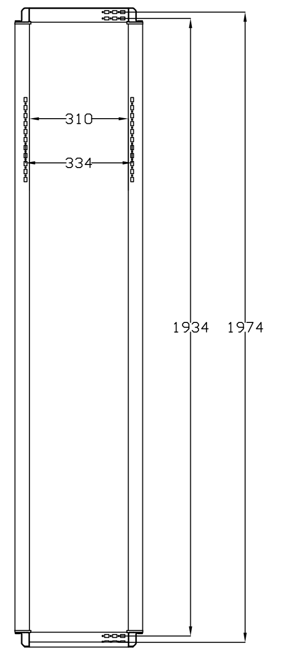
SEC. A-A
