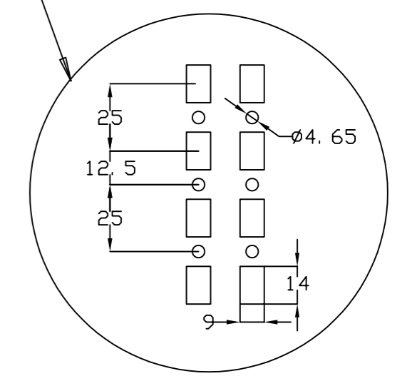
DETALLE DEL PERFIL PROFILE DETAIL
