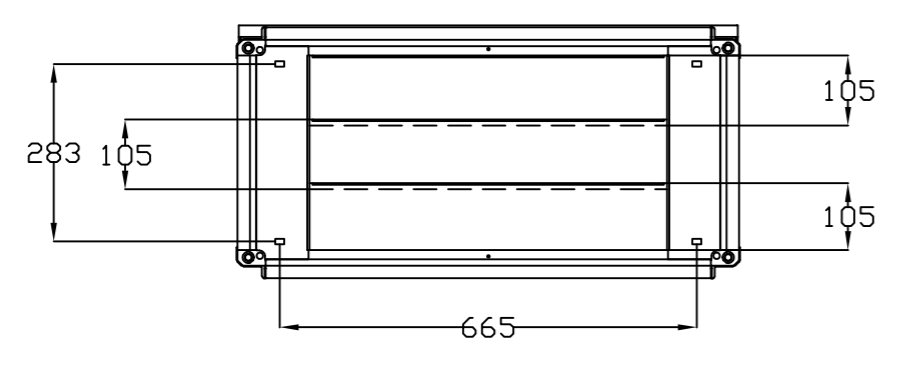
VISTA INFERIOR BOTTOM VIEW
