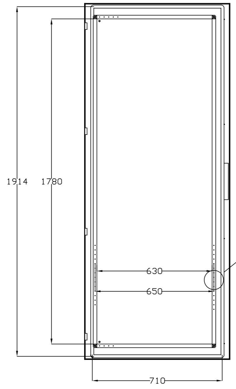
VISTA POSTERIOR PUERTA DOOR REAR VIEW
