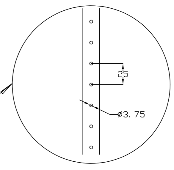
DETALLE DEL REFUERZO PROFILE DETAIL
