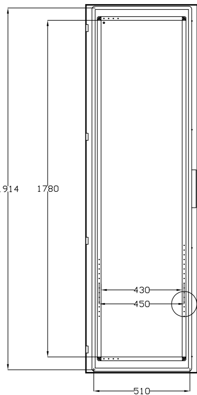
VISTA POSTERIOR PUERTA DOOR REAR VIEW
