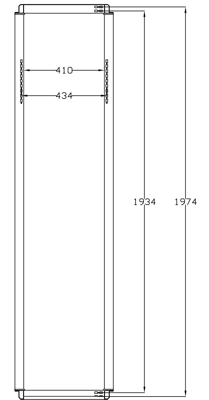
SEC. A-A
