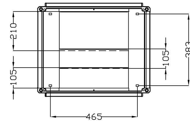
VISTA INFERIOR BOTTOM VIEW
