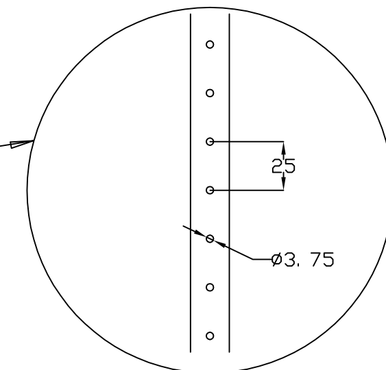
DETALLE DEL REFUERZO PROFILE DETAIL
