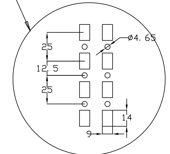
DETALLE DEL PERFIL PROFILE DETAIL
