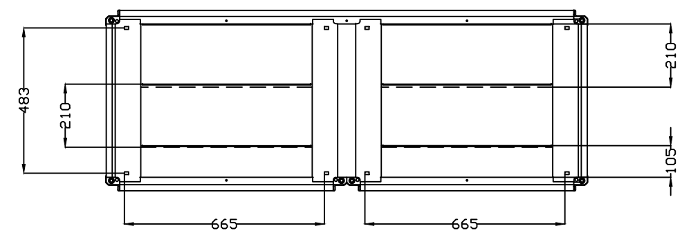
VISTA INFERIOR BOTTOM VIEW
