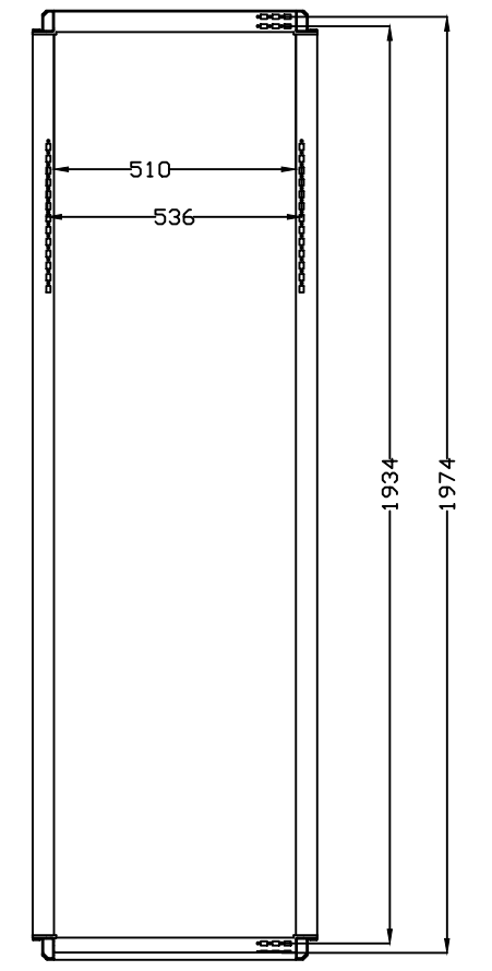
SEC. A-A
