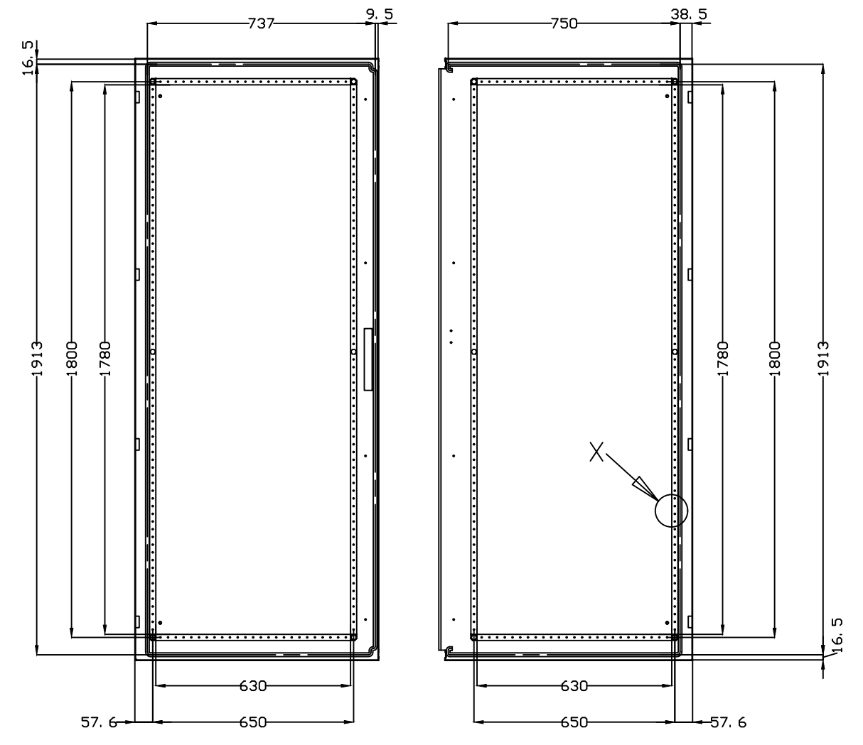
VISTA POSTERIOR PUERTA DOOR REAR VIEW
