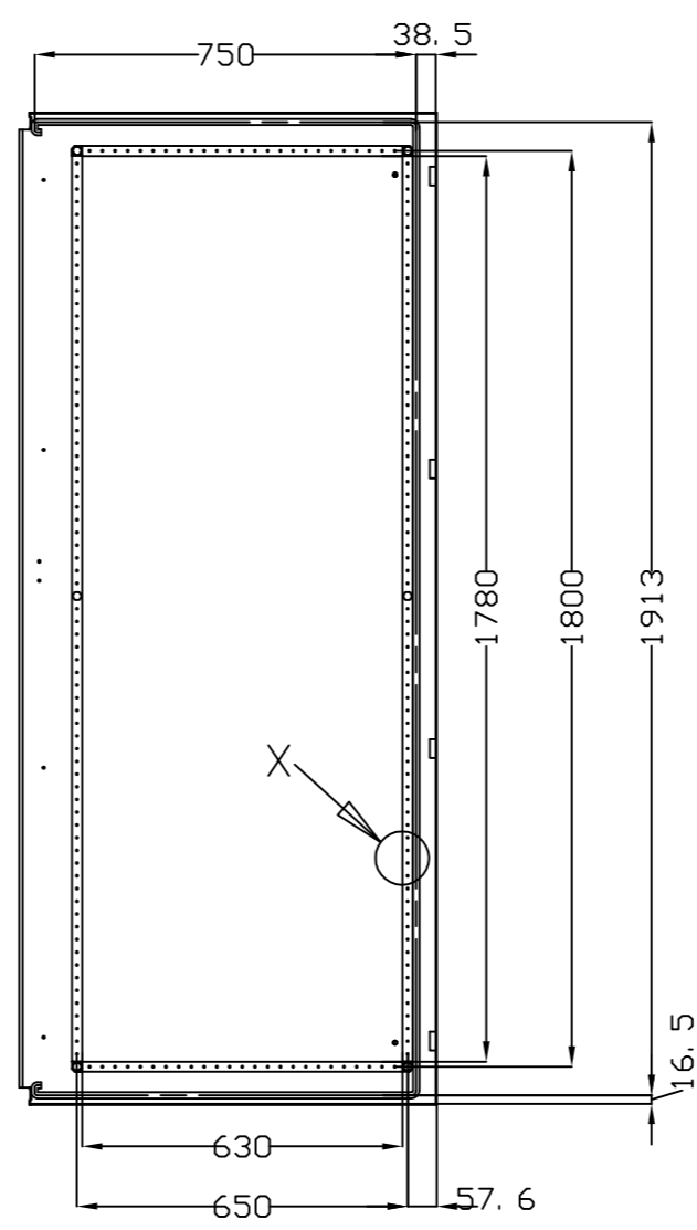
VISTA POSTERIOR PUERTA DOOR REAR VIEW
