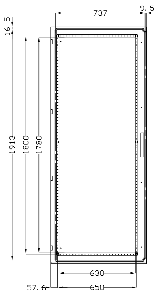
VISTA POSTERIOR PUERTA DOOR REAR VIEW
