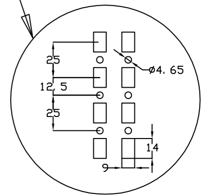
DETALLE DEL PERFIL PROFILE DETAIL
