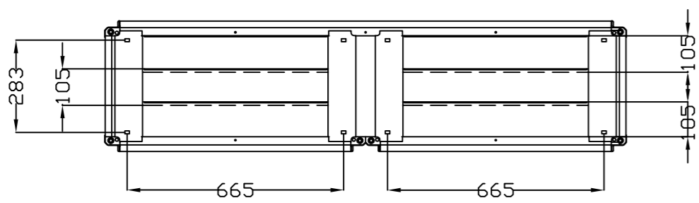
VISTA INFERIOR BOTTOM VIEW
