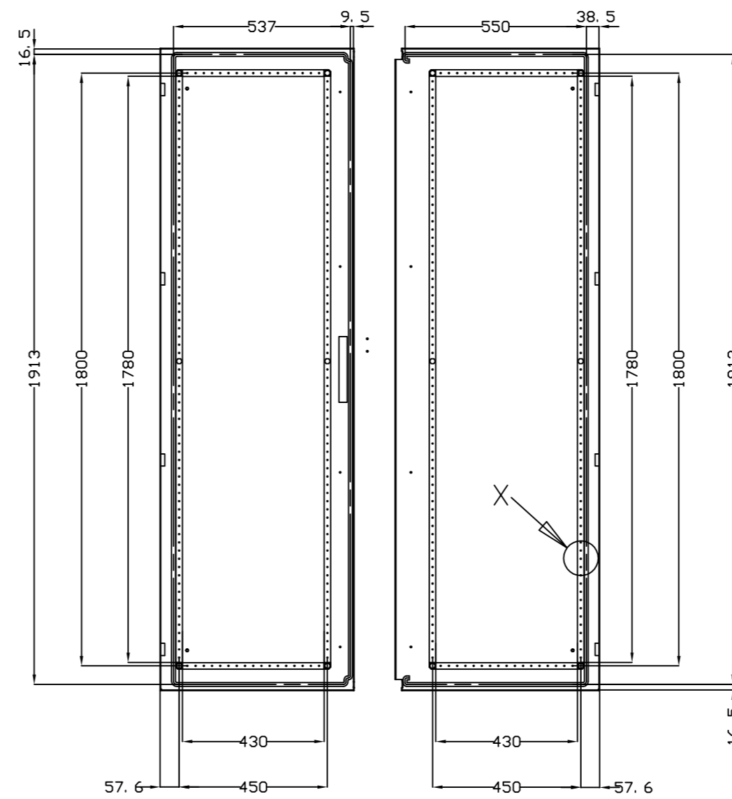
VISTA POSTERIOR PUERTA DOOR REAR VIEW
