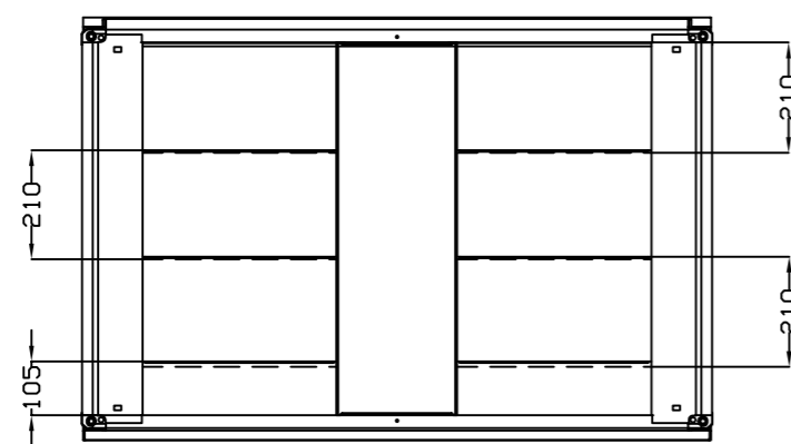
VISTA INFERIOR BOTTOM VIEW
