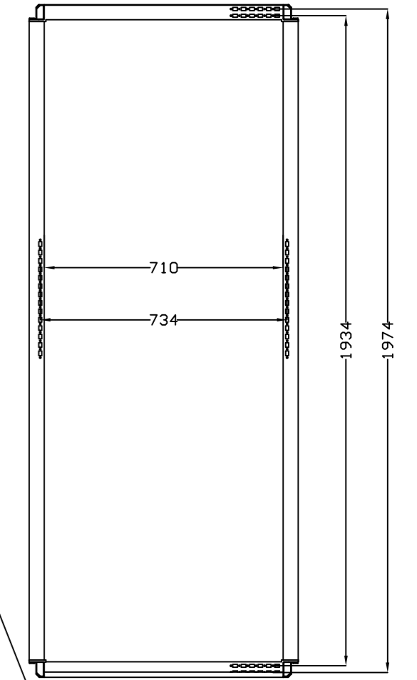
SEC. A-A
