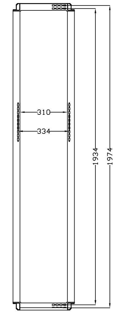
SEC. A-A
