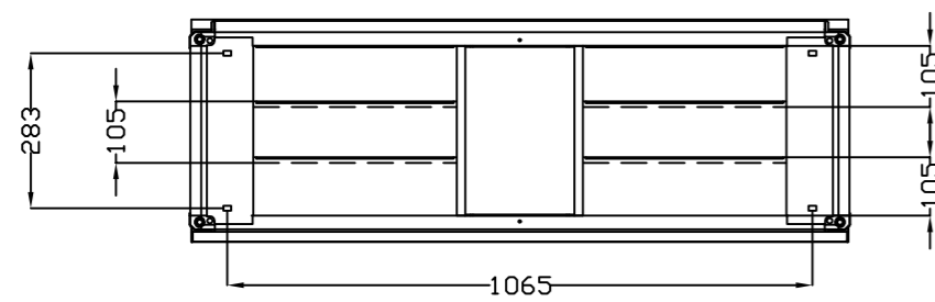
VISTA INFERIOR BOTTOM VIEW
