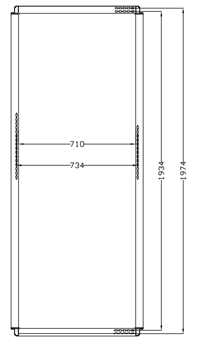
SEC. A-A
