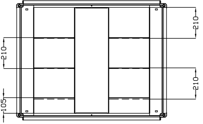
VISTA INFERIOR BOTTOM VIEW
