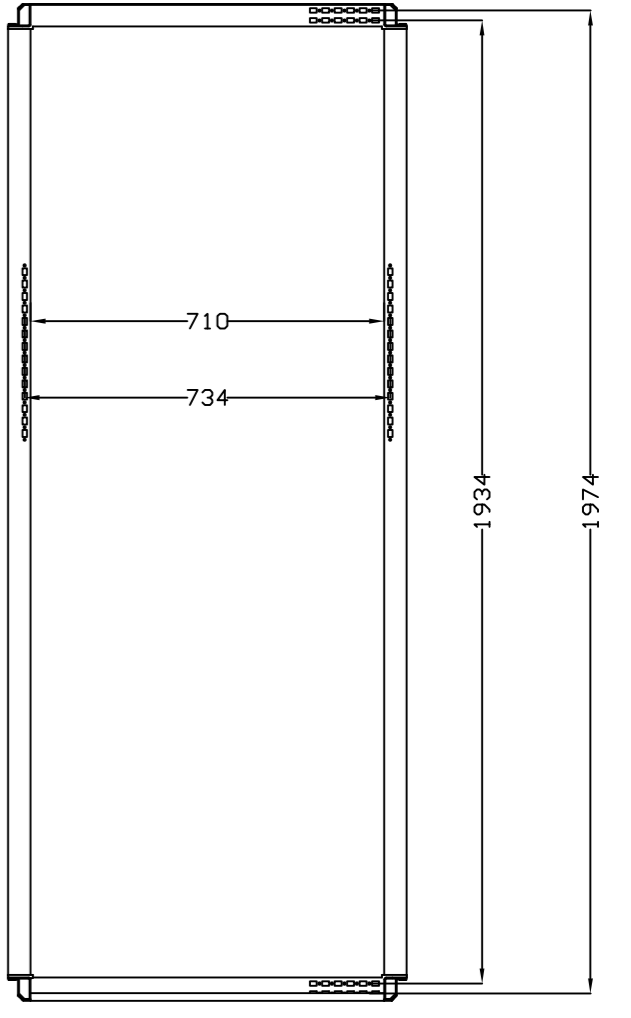
SEC. A-A
