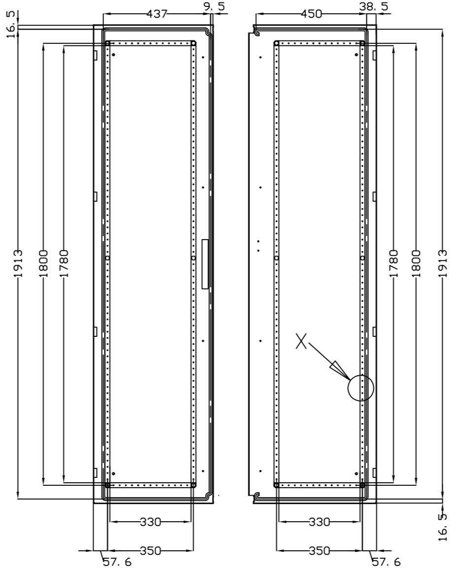
VISTA POSTERIOR PUERTA DOOR REAR VIEW
