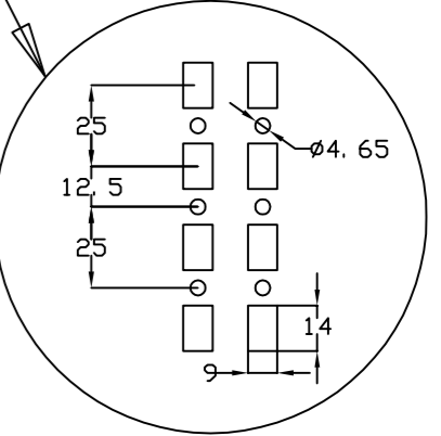
DETALLE DEL PERFIL PROFILE DETAIL
