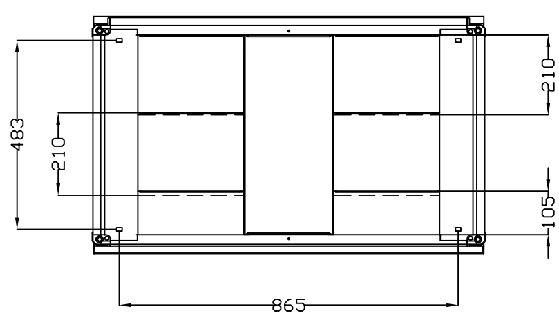
VISTA INFERIOR BOTTOM VIEW
