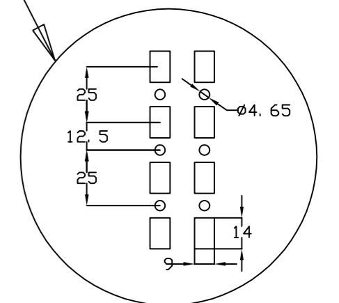
DETALLE DEL PERFIL PROFILE DETAIL
