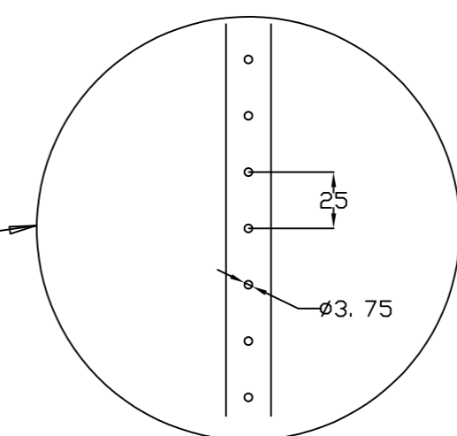
DETALLE DEL REFUERZO PROFILE DETAIL
