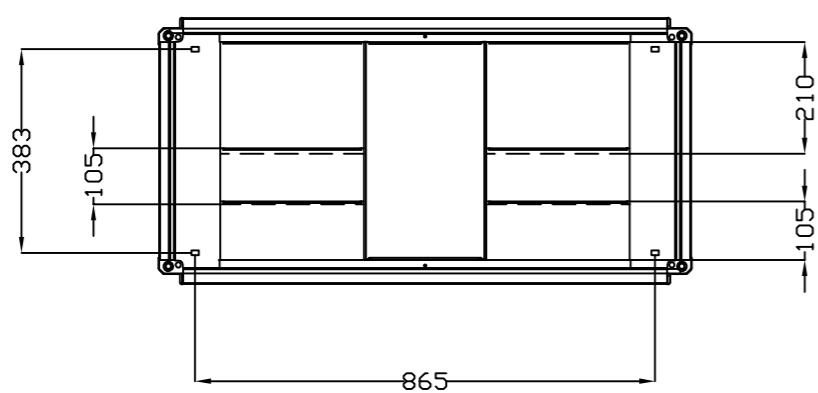
VISTA INFERIOR BOTTOM VIEW
