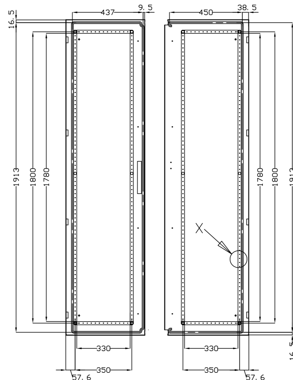
VISTA POSTERIOR PUERTA DOOR REAR VIEW
