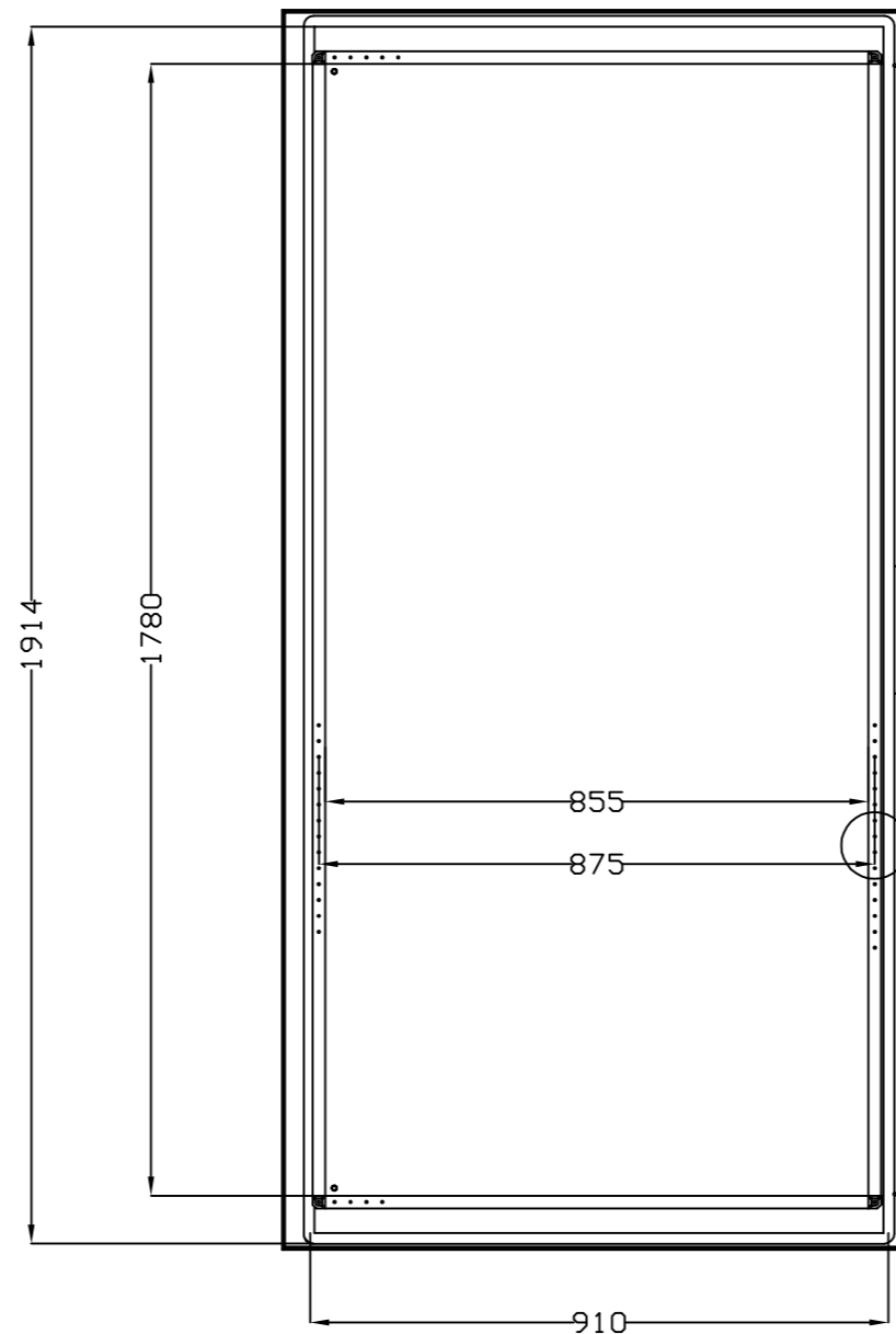
VISTA POSTERIOR PUERTA DOOR REAR VIEW
