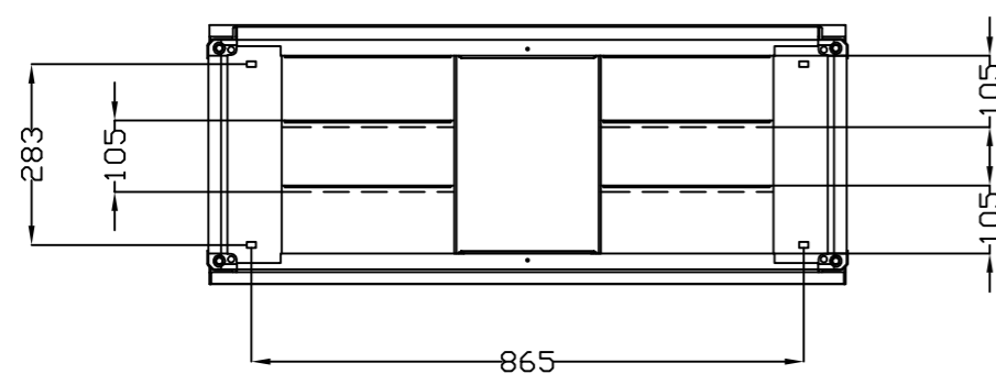
VISTA INFERIOR BOTTOM VIEW
