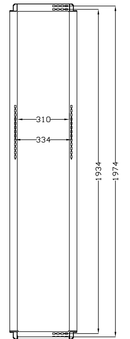
SEC. A-A
