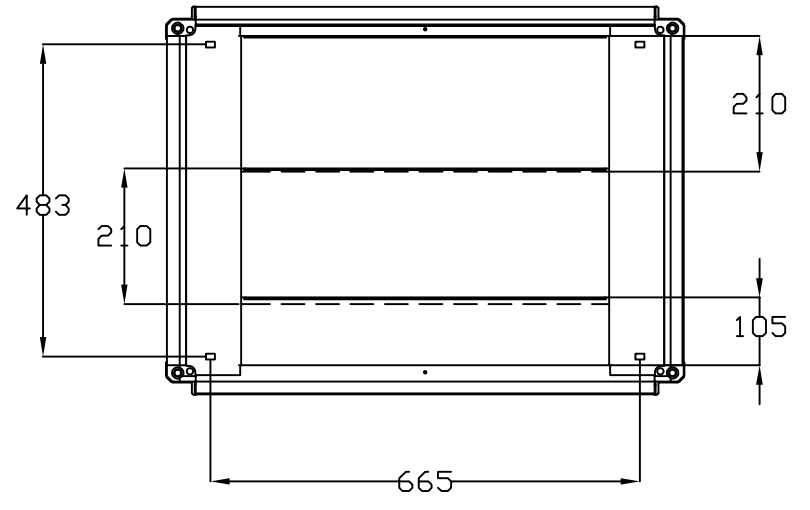
VISTA INFERIOR BOTTOM VIEW
