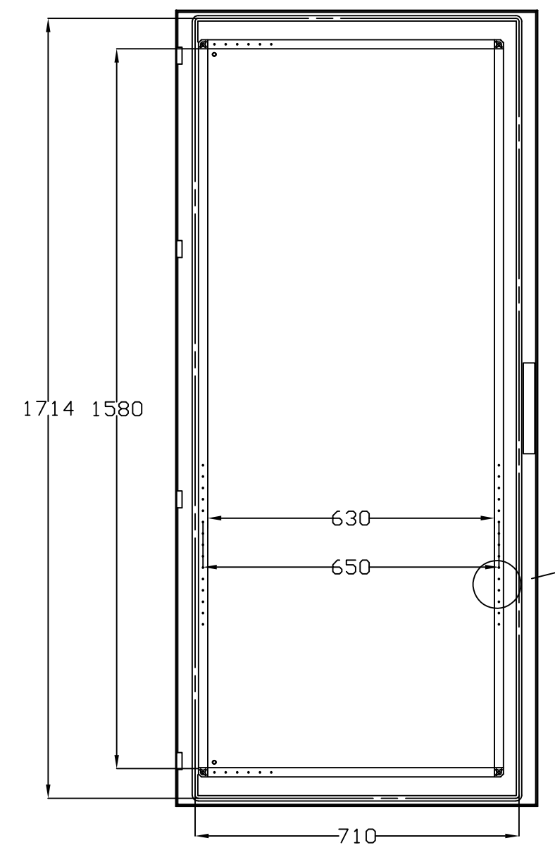
VISTA POSTERIOR PUERTA DOOR REAR VIEW
