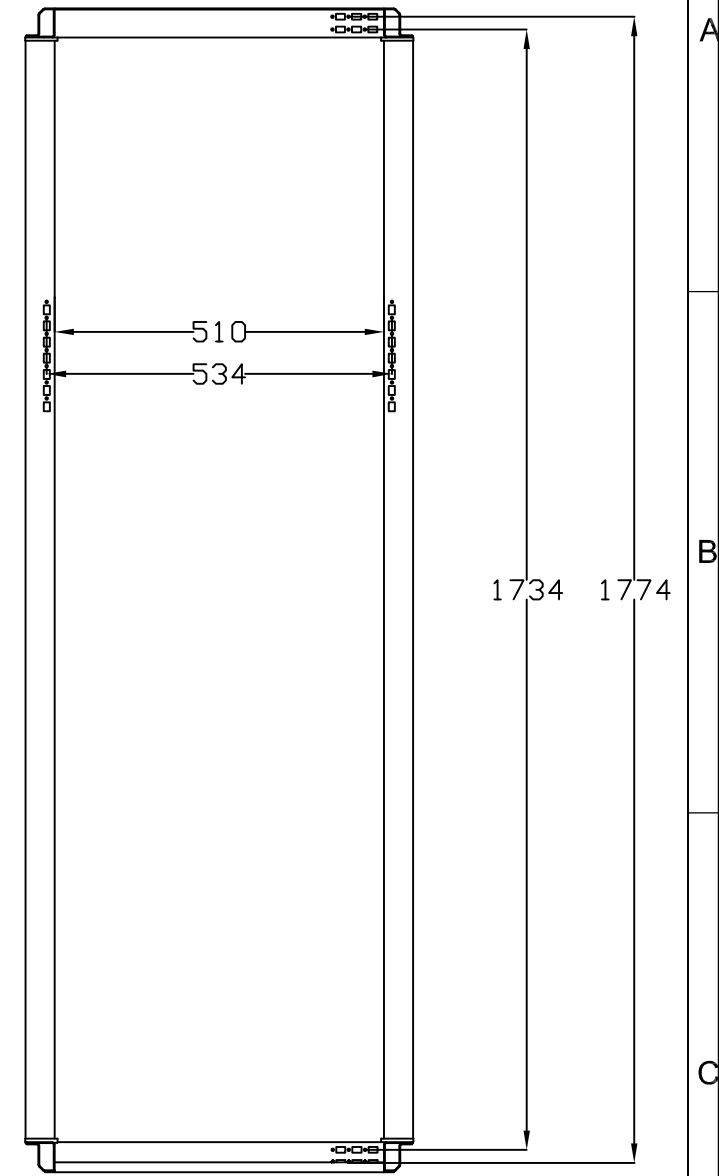
SEC. A-A
