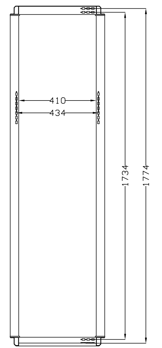
SEC. A-A
