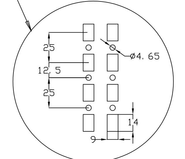
DETALLE DEL PERFIL PROFILE DETAIL
