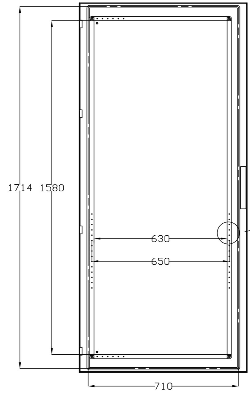
VISTA POSTERIOR PUERTA DOOR REAR VIEW
