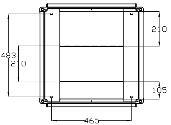
VISTA INFERIOR BOTTOM VIEW
