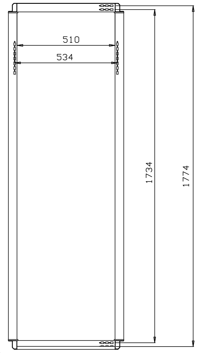
SEC. A-A
