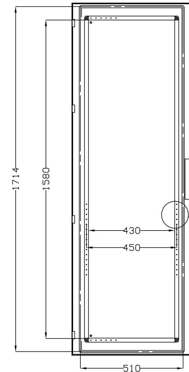
VISTA POSTERIOR PUERTA DOOR REAR VIEW
