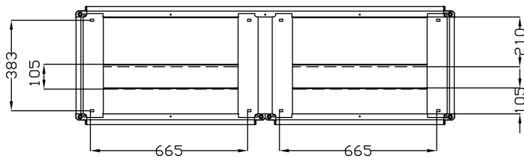
VISTA INFERIOR BOTTOM VIEW
