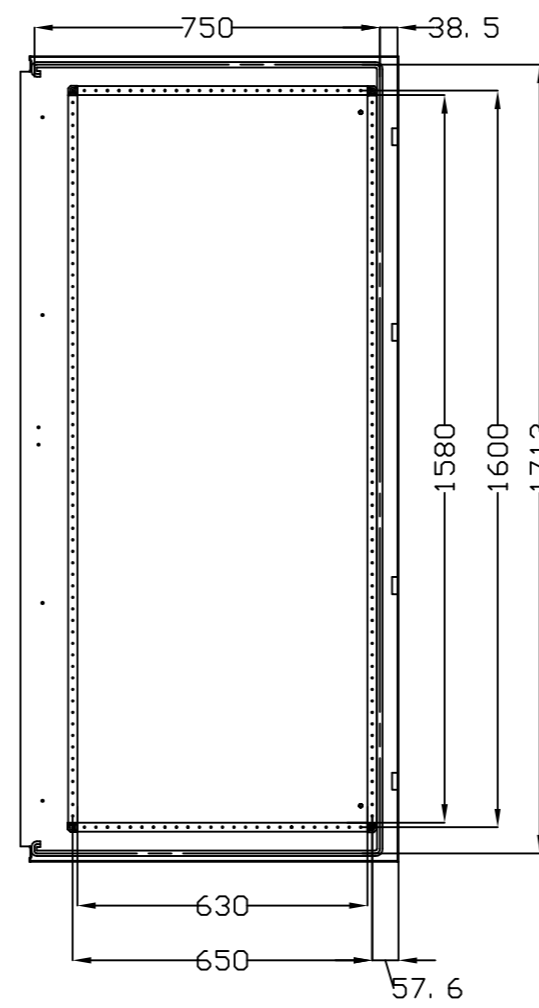
VISTA POSTERIOR PUERTA DOOR REAR VIEW
