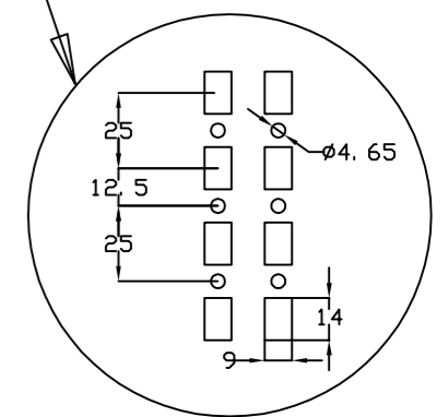
DETALLE DEL PERFIL PROFILE DETAIL
