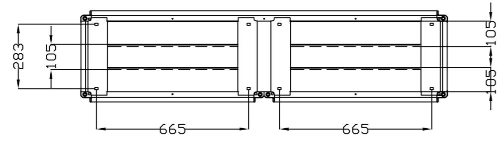
VISTA INFERIOR BOTTOM VIEW
