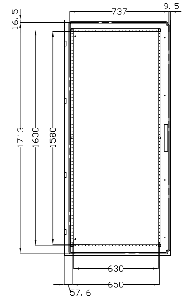
VISTA POSTERIOR PUERTA DOOR REAR VIEW
