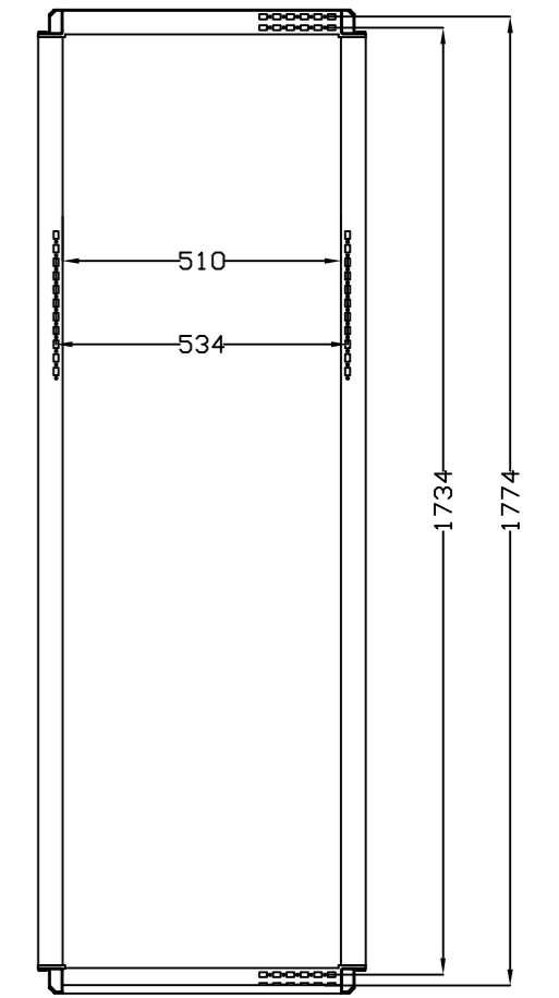
SEC. A-A
