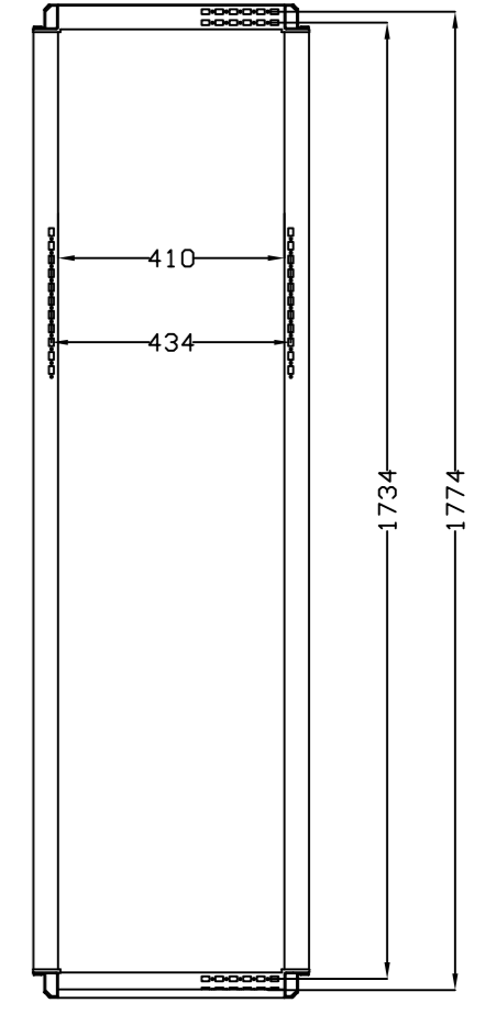
SEC. A-A
