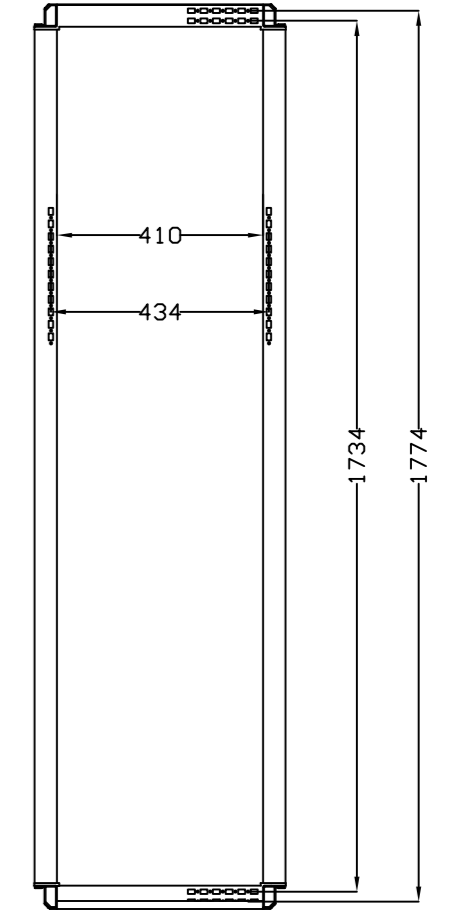
SEC. A-A
