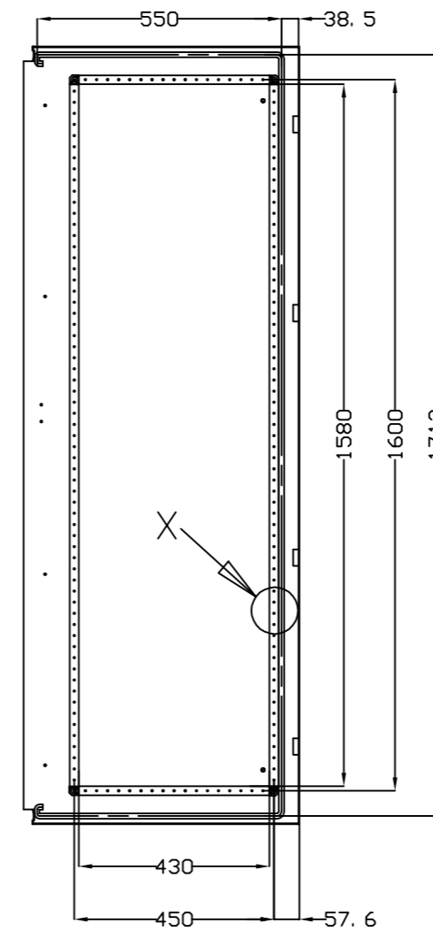
VISTA POSTERIOR PUERTA DOOR REAR VIEW
