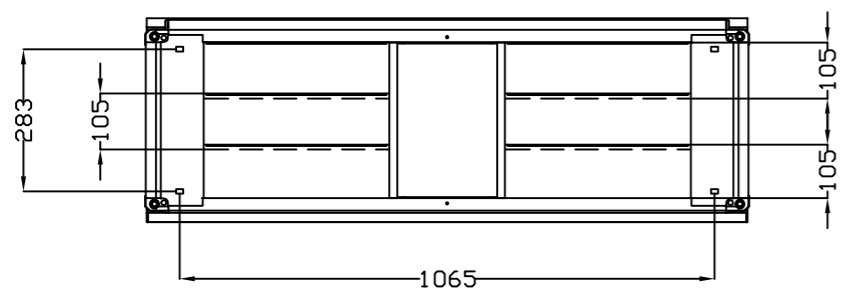
VISTA INFERIOR BOTTOM VIEW
