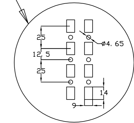
DETALLE DEL PERFIL PROFILE DETAIL
