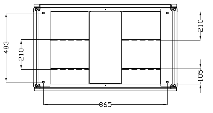
VISTA INFERIOR BOTTOM VIEW
