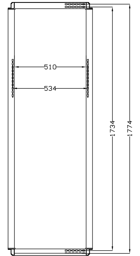
SEC. A-A
