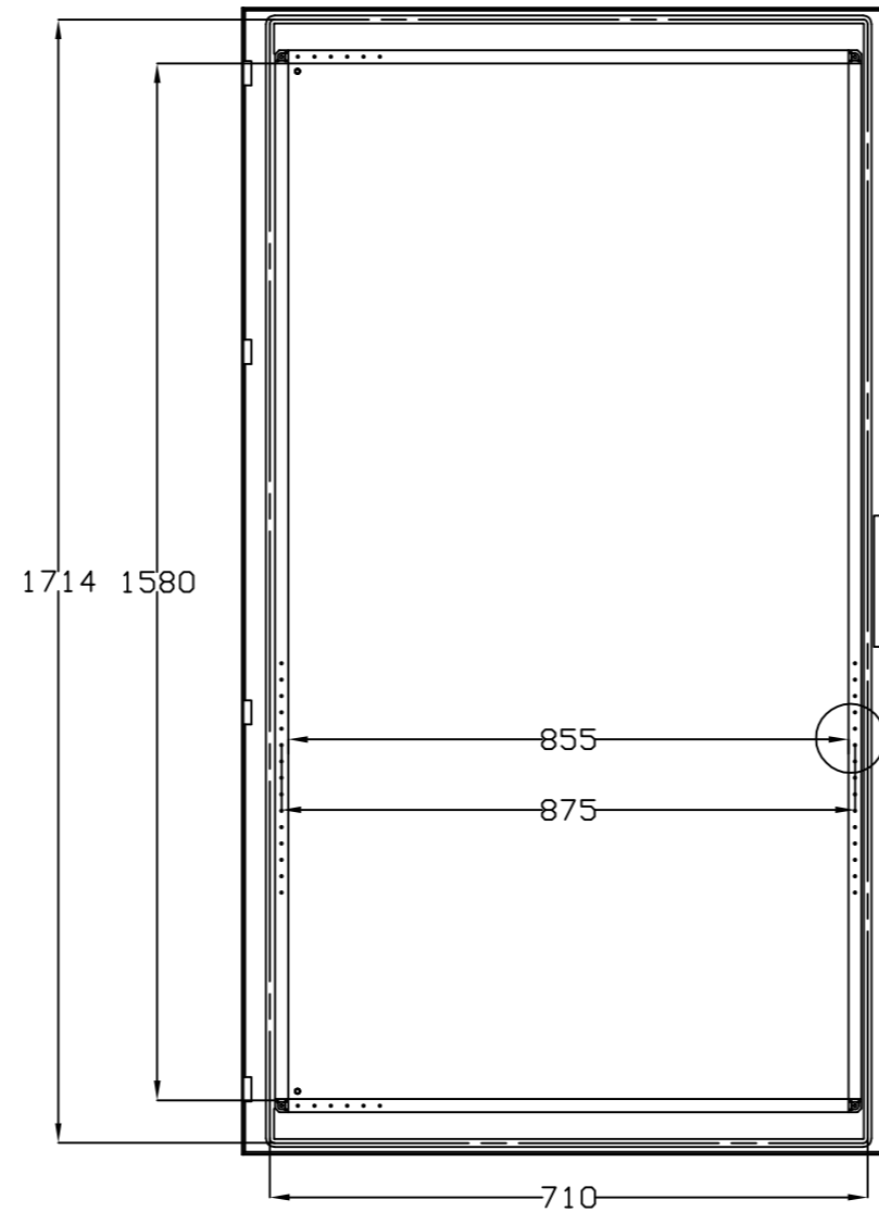
VISTA POSTERIOR PUERTA DOOR REAR VIEW
