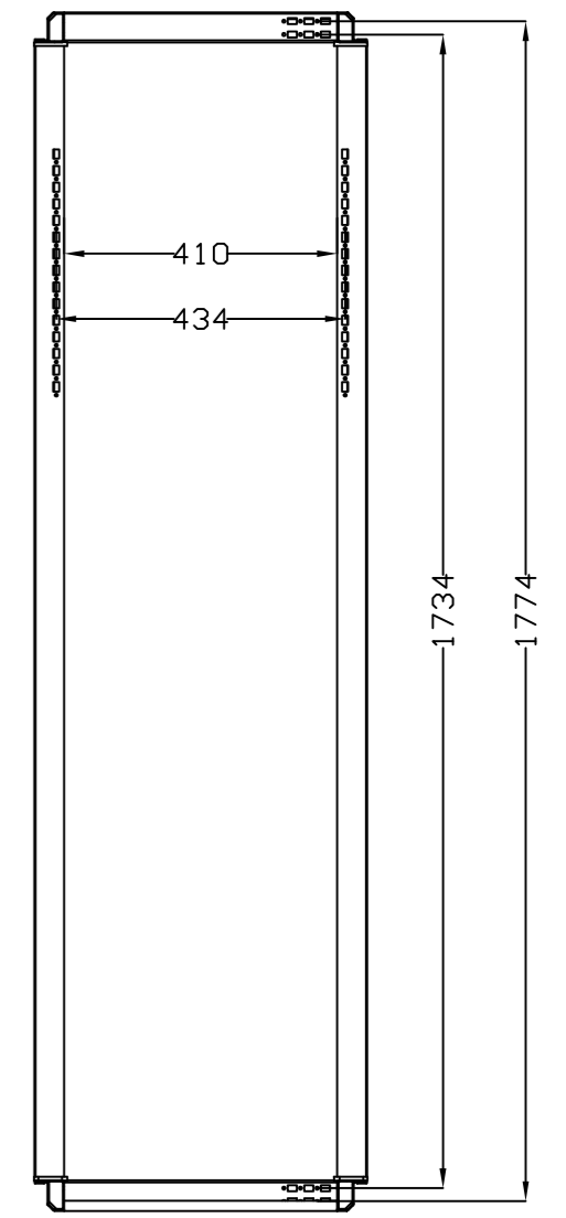
SEC. A-A
