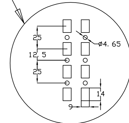
DETALLE DEL PERFIL PROFILE DETAIL
