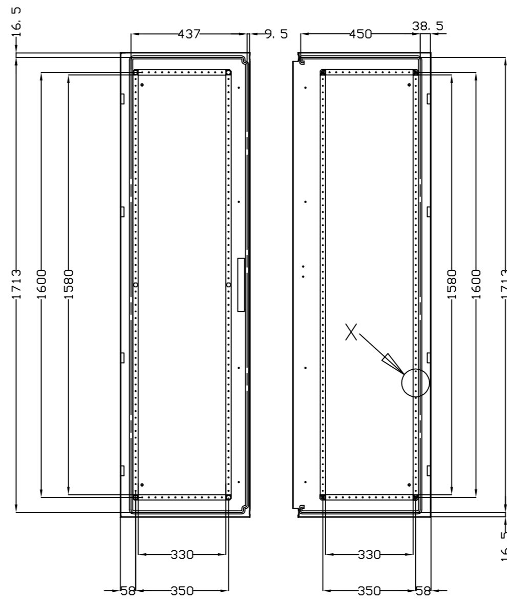
VISTA POSTERIOR PUERTA DOOR REAR VIEW
