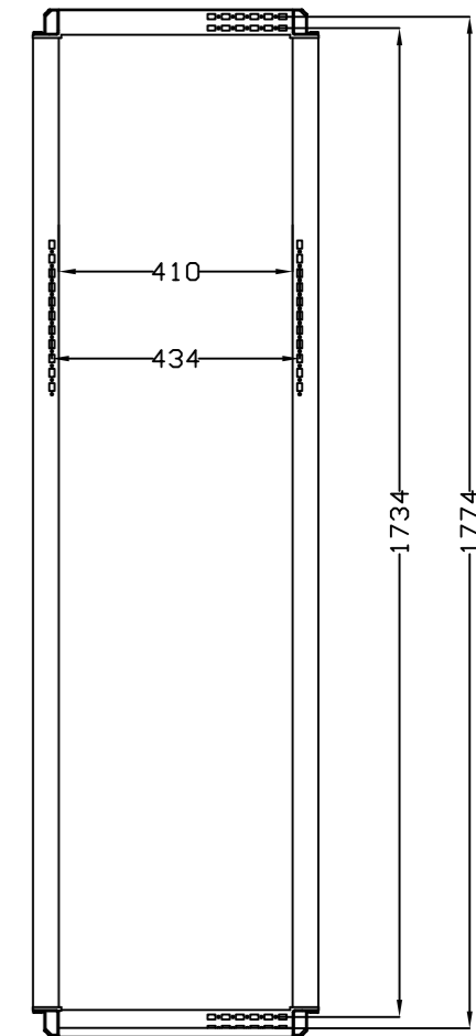
SEC. A-A
